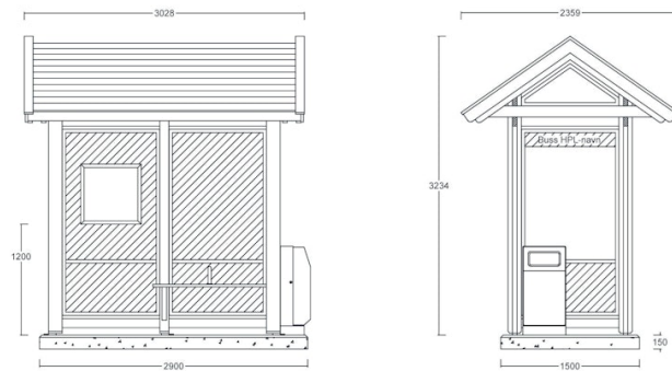
1120 011 Tremiljø Rapid RSCEE (2 felt) 3028 x 2359 mm
