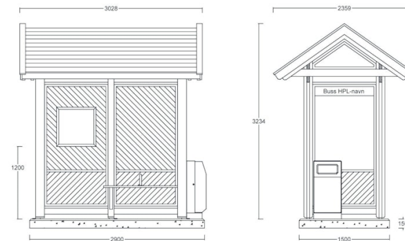
1120 012 Tremiljø Rapid RSCEE (2 felt) 3028 x 2359 mm
