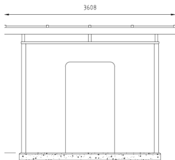
1304 City 90 Traffic ladestasjon (1 modul) Ø90 stolpe, for 0 x 0 025 1 lader mm
